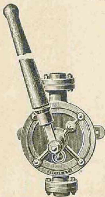
Pompes demi-rotatives à double ou quadruple effet 9 tailles dans 5 dispositions
